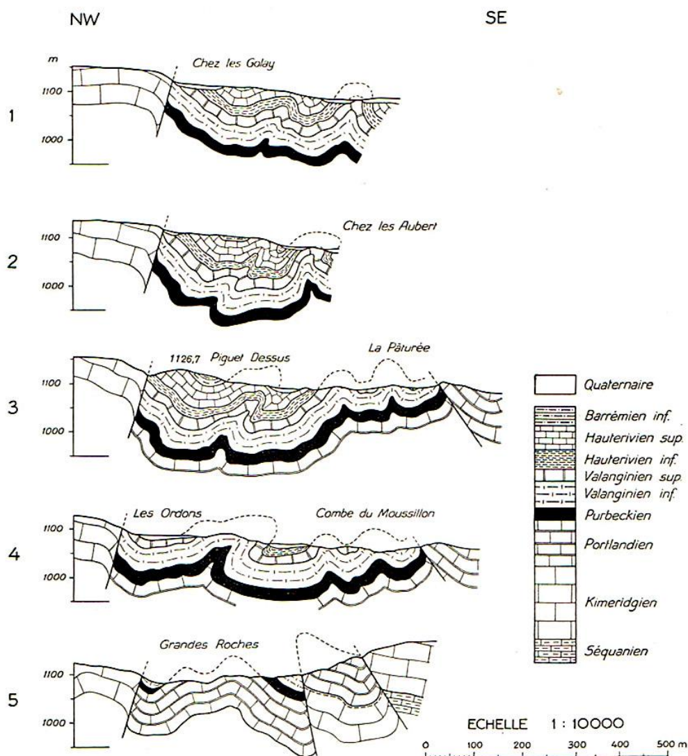
Fig. 20. Coupes tectoniques de la région des Piguet Dessus.
