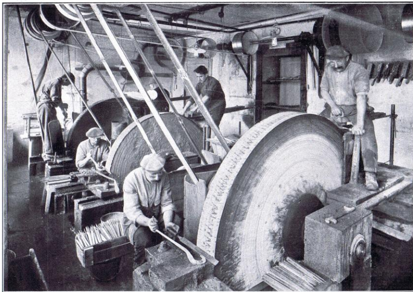
Fig. 9. — Un atelier du meulage des limes.
