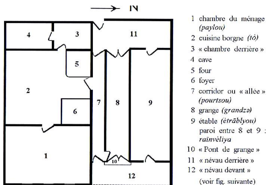
fig. 10 Plan d'une ferme ancienne (dimensions 20 × 20 m)
