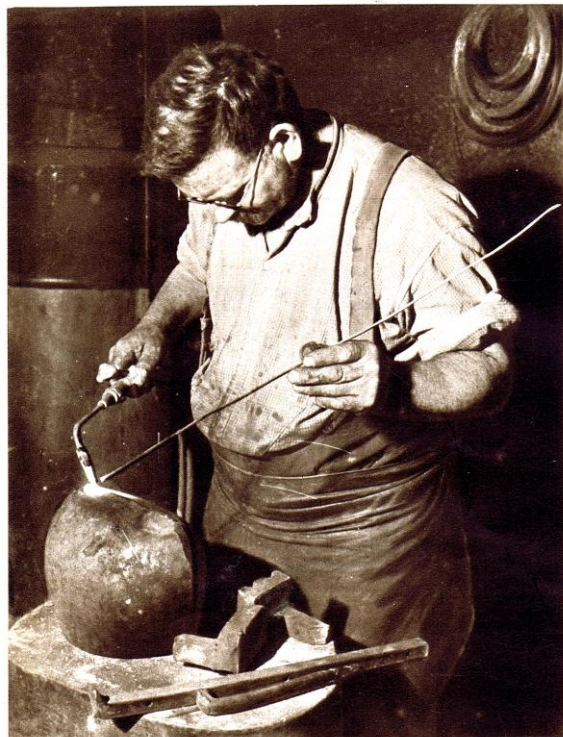
Montage et soudure à l'autogène de la partie supérieure de la sonnette, à laquelle sont fixés ensuite le porte-courroie et le porte-battant.
