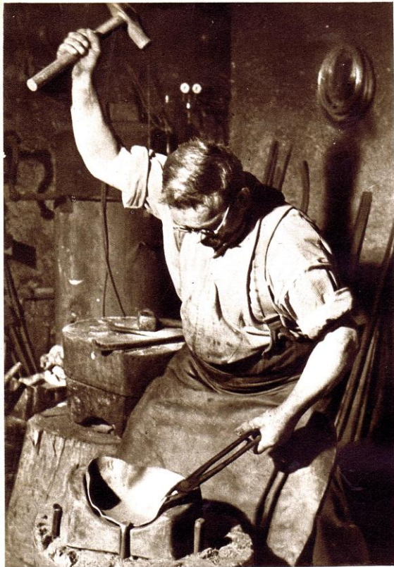
A grands coups de marteau, le planage dans la forme de fonte, dont la grandeur varie suivant le numéro de la sonnette.
